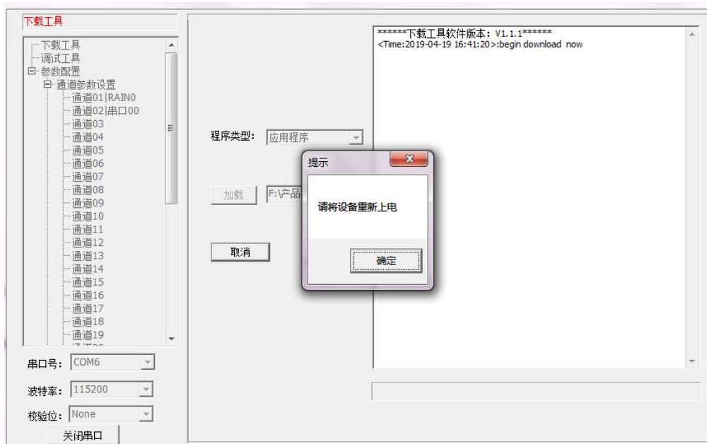
步骤 3. RTU 设备重新上电，程序开始升级
